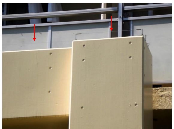
都営住宅 耐震改修工事 (コンクリート打ちタイプ)
