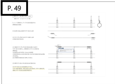
F-2 支柱 UBS-P Φ1.2 UBW□-ール + UBW(B)グリップ
