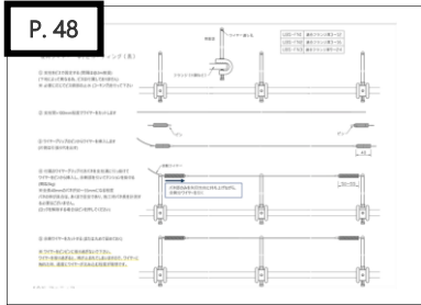
D-2 支柱 UBS-FN Φ1.2 UBW□-ール + UBW(B)グリップ
